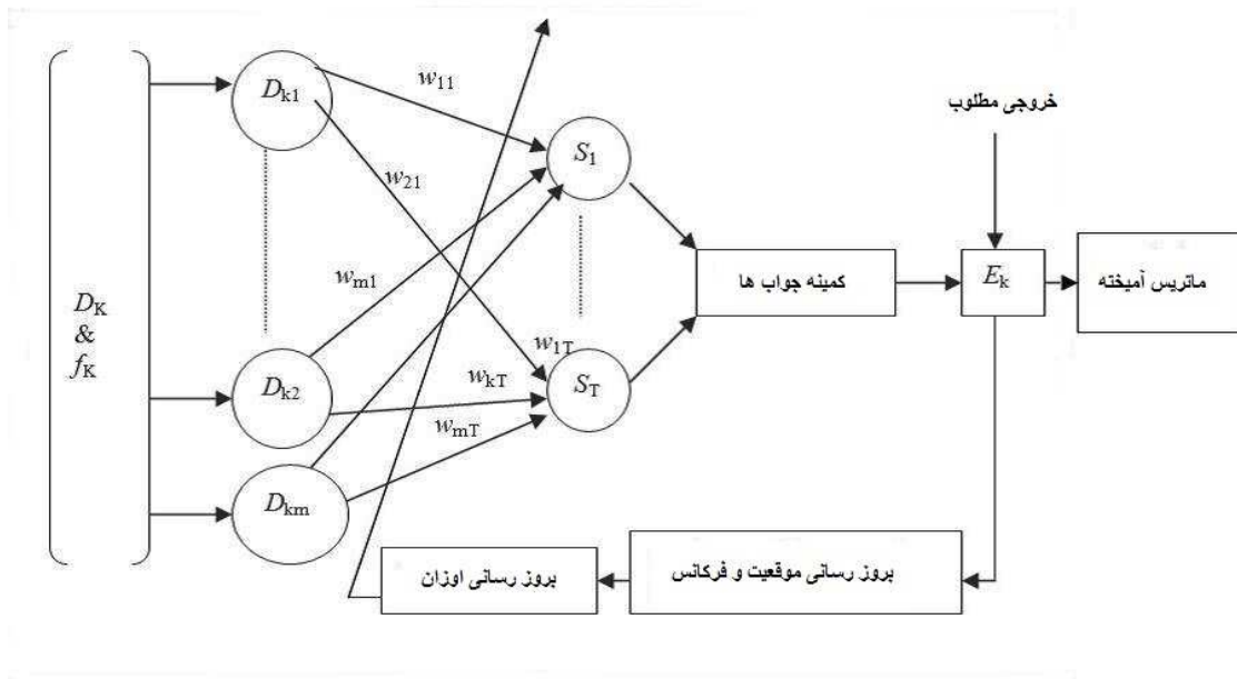
شکل ۴. الگوریتم بت
