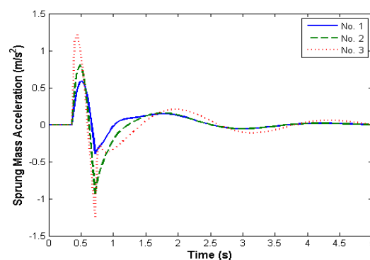
شکل ۱۵. نمودار شتاب جرم فربندی شده بر حسب زمان؛ بهینه شده توسط روش الگوریتم ژنتیک در ۳ نقطه طراحی مختلف
