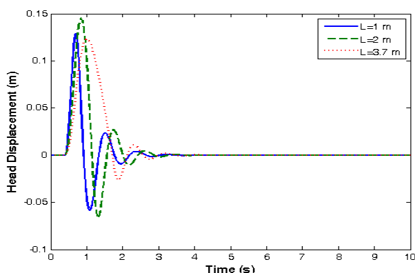
شکل ۸. نمودار جابه‌جایی سر راننده بر حسب زمان در حالت بهینه نشده و در پهنای دست‌انداز متفاوت
