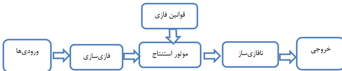
شکل ۱. مدل‌سازی فازی
