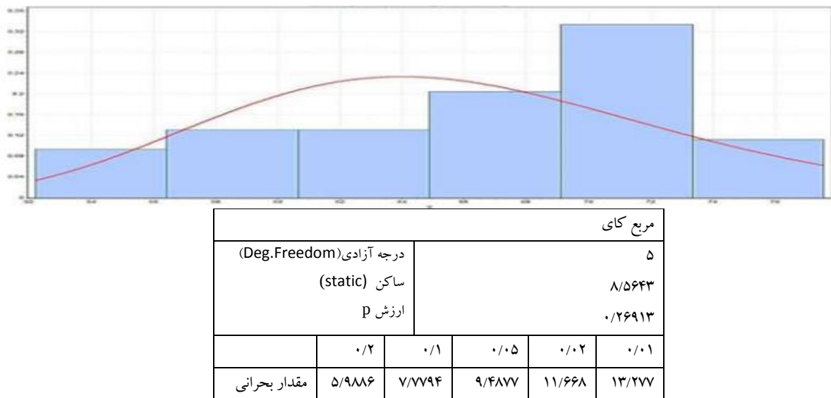
شکل ۷. نمودار توزیع مربع کای برای جنگل تصادفی
