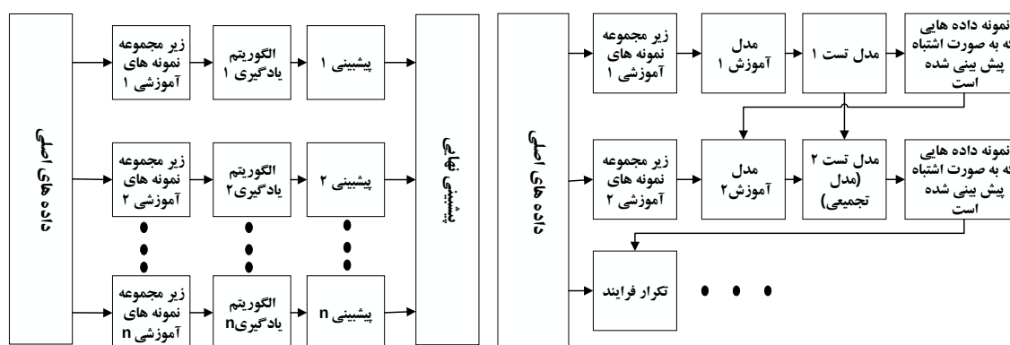
شکل ۴. دیاگرام یادگیری دسته‌بندی تقویتی (سمت راست) و دسته‌ای (سمت چپ)
