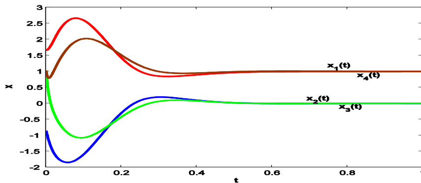
شکل ۳. رفتارهای گذرای x_1 ، x_2 ، x_3 و x_4 از شبکه عصبی (۱۶) در مثال (۳-۶).
