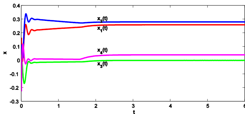
شکل ۴. رفتارهای گذرای x_1 ، x_2 ، x_3 و x_4 از شبکه عصبی (۱۶) در مثال (۴-۶).
