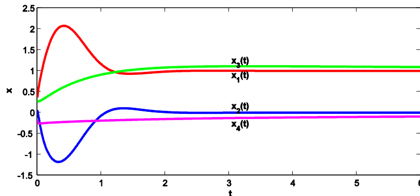
شکل ۵. رفتارهای گذرای x_1 ، x_2 ، x_3 و x_4 از شبکه عصبی (۱۶) در مثال (۵-۶).
