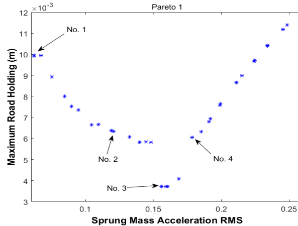
شکل ۱۷. نمودار پارتو مربوط به دو تابع هدف RMS شتاب جرم فنربندی شده و اختلاف جابجایی تایر و ورودی سطح جاده
