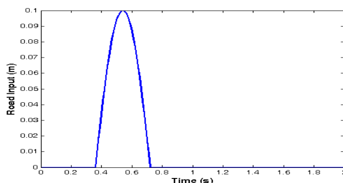
شکل ۳. ورودی جاده به سیستم تعلیق خودرو به ازای دست‌انداز با طول ۱ متر [۲۴]
