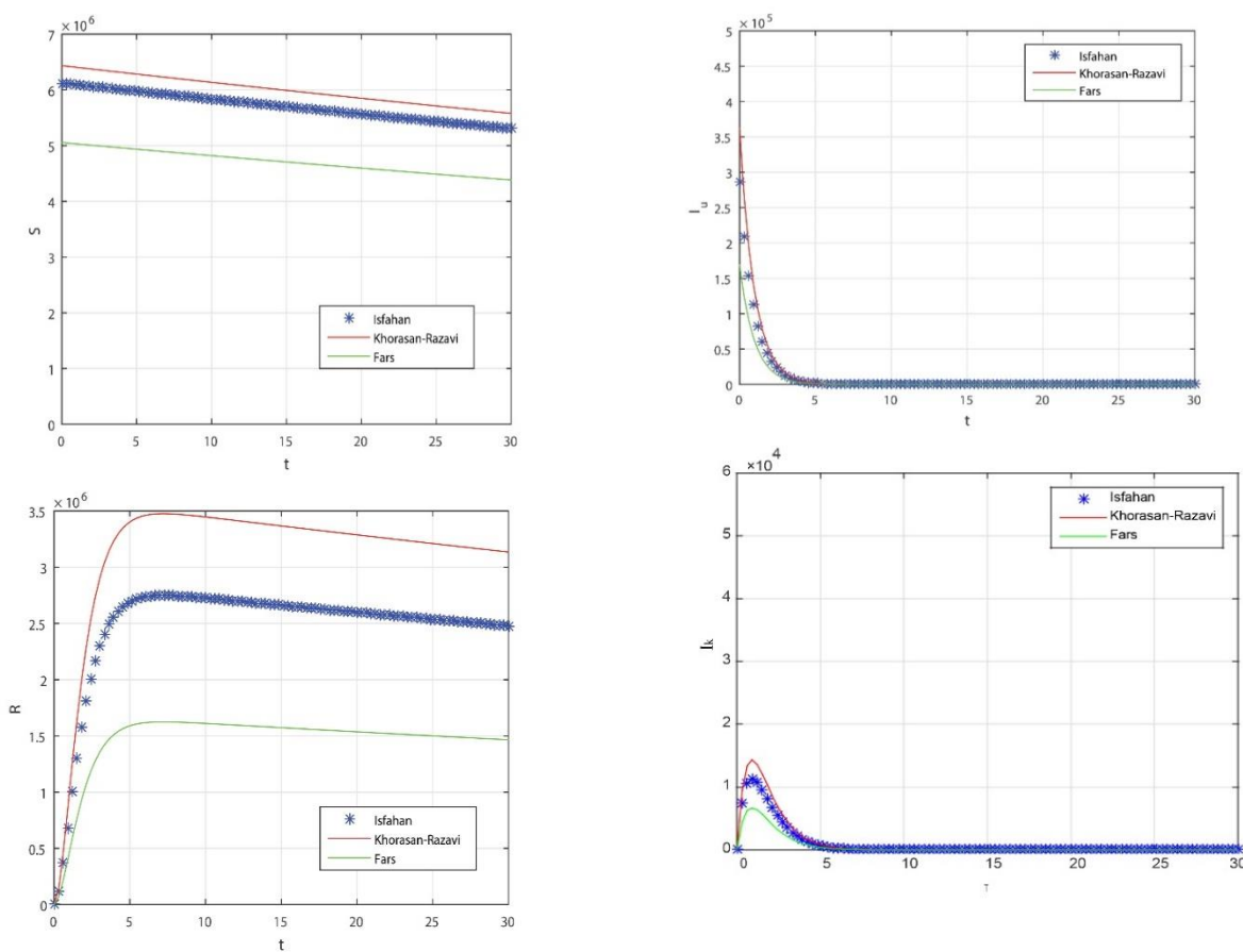
شکل ۴. نمودارهای S ، I_k ، I_u و R در سه استان با کنترل با استفاده از داده‌های جدول ۲
