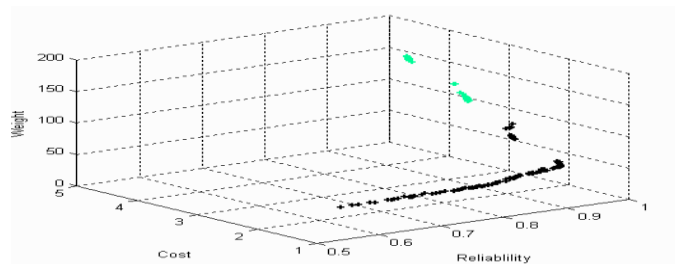
شکل ۹. خوشه‌بندی جواب‌های بهینه پارتو در حالت Reliability-cost-weight
