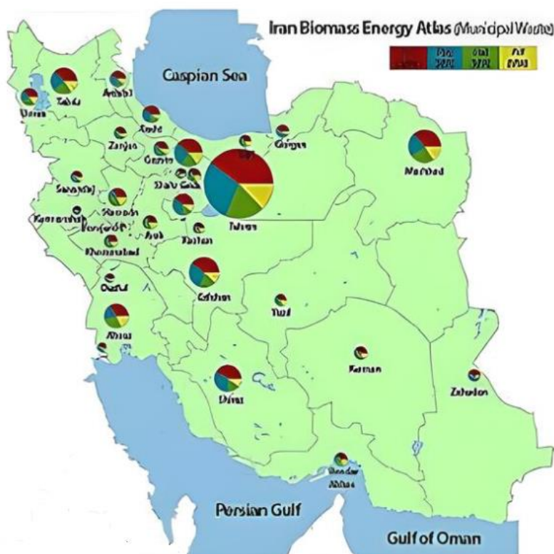
شکل ۳. پراکندگی منابع زیست توده در ایران
