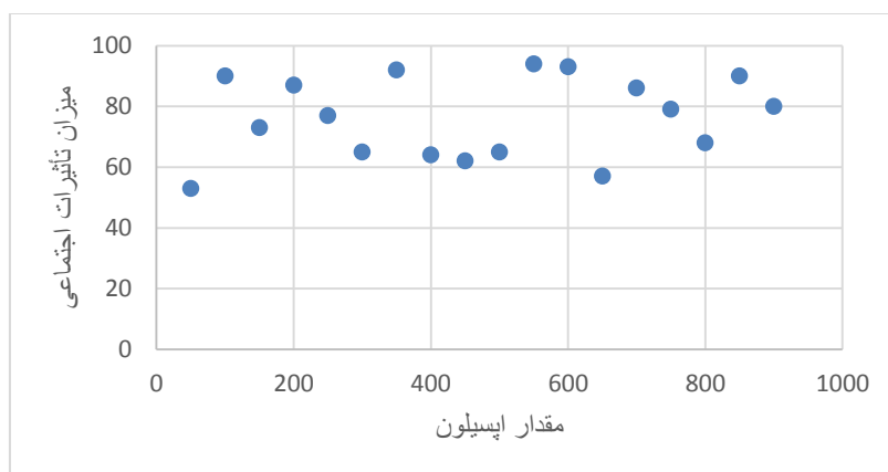
شکل ۷. میزان تغییرات تأثیرات اجتماعی به ازای تغییرات ایزوپروپیلون
