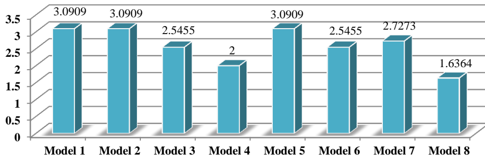
شکل ۱. اختلاف رتبه مدل‌ها با روش IIEP - DEA
