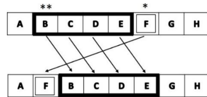
شکل ۴. جهش الحاقی
