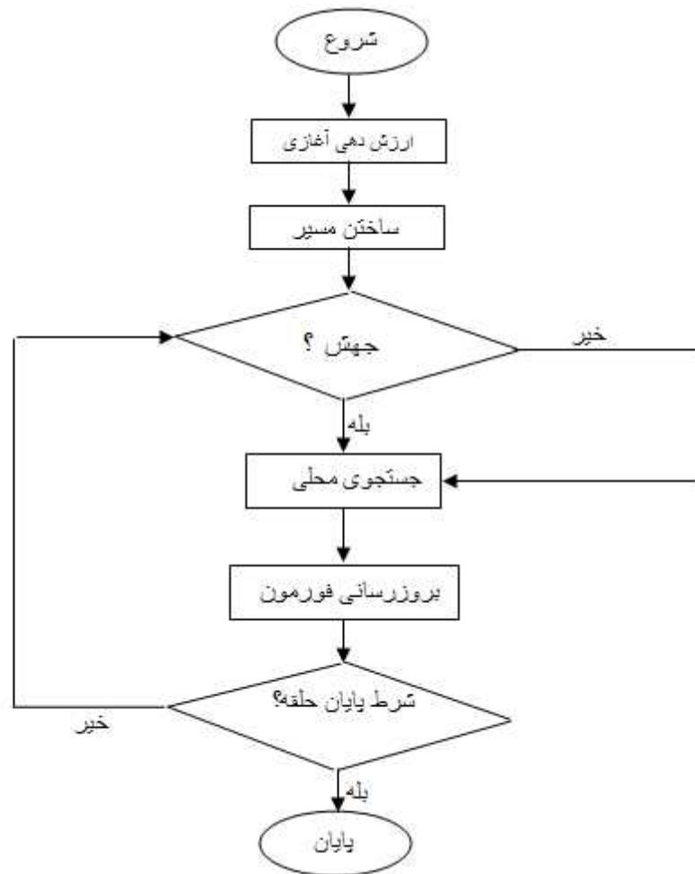
شکل ۲. فلوچارت الگوریتم پیشنهادی
