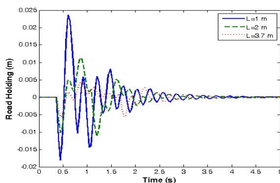
شکل ۶. نمودار اختلاف ورودی جاده و تایر بر حسب زمان در حالت بهینه نشده و با پهنای دست‌انداز متفاوت
