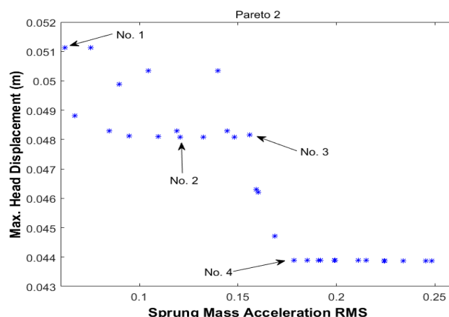
شکل ۱۸. نمودار پارتو مربوط به دو تابع هدف RMS شتاب جرم فربندی شده و جابجایی سر راننده
