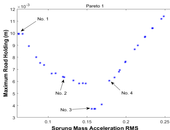
شکل ۱۷. نمودار پارتو مربوط به دو تابع هدف RMS شتاب جرم فربندی شده و اختلاف جابجایی تایر و ورودی سطح جاده
