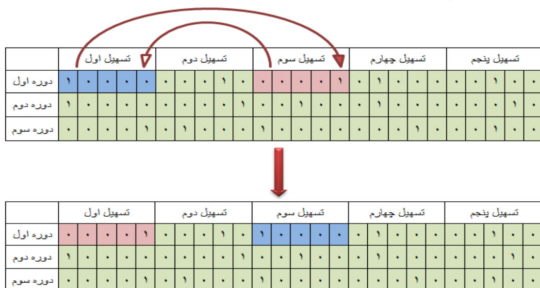
شکل ۴. چگونگی ایجاد ساختار همسایگی در الگوریتم شبیه‌ساز تبرید موازی
