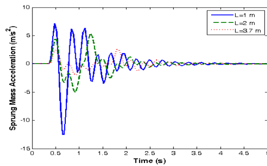
شکل ۷. نمودار شتاب جرم فنر بندی شده بر حسب زمان در حالت بهینه نشده و با پهنای دست‌انداز متفاوت
