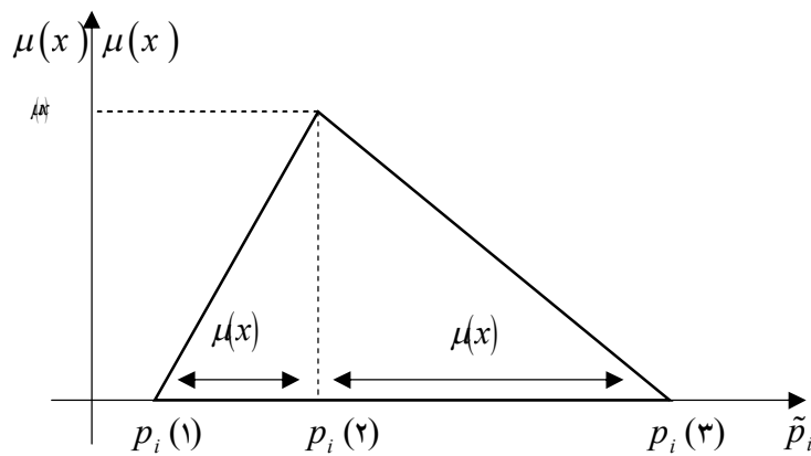
شکل ۲. توزیع امکانی عدد فازی مثلثی
